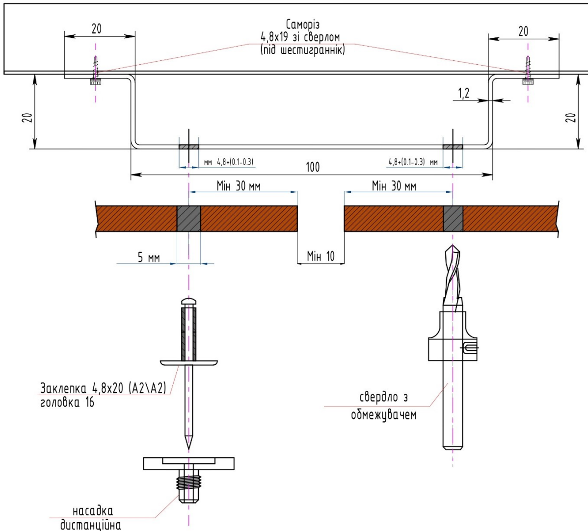
Схема кріплення листів Вид зверху
