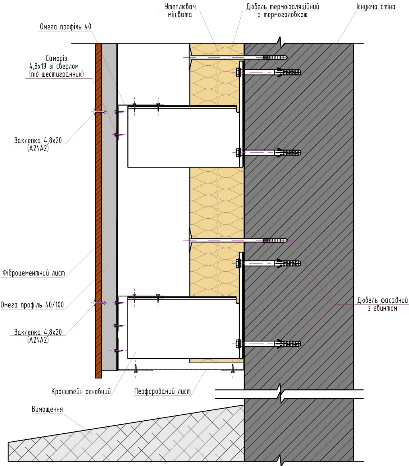
Схема кріплення фіброцементних листів на цокольній частині (варіант 1)
